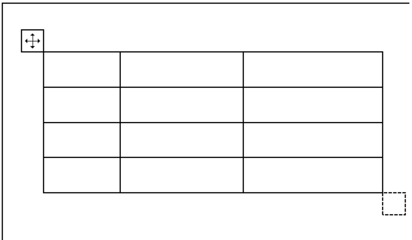
Abbildung: Griff
