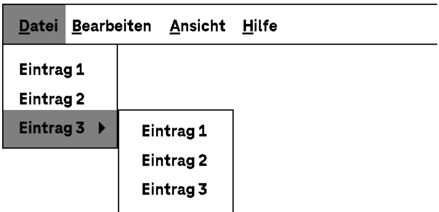
Abbildung: Anwendungsmenü
