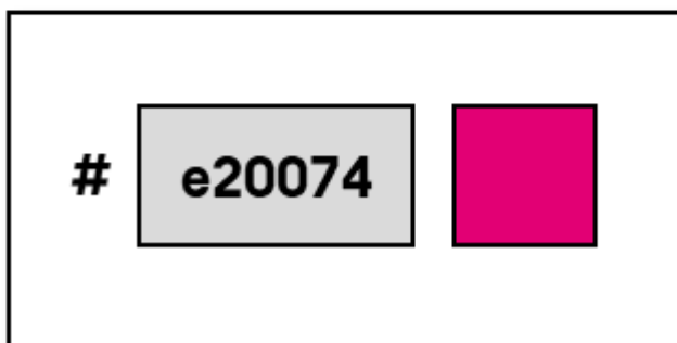
Abbildung: Farbwähler
