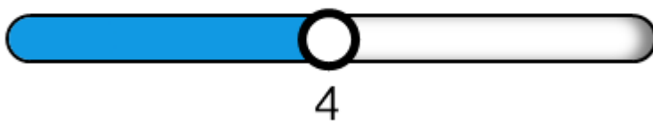
Abbildung: Schieberegler
