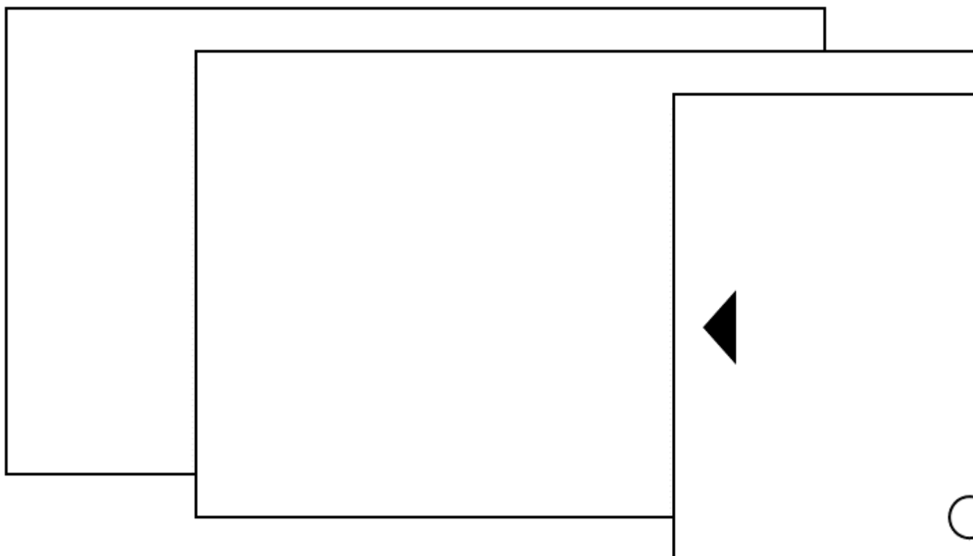
Abbildung: Karussell
