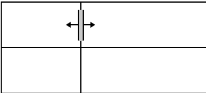
Abbildung: Bereichstrenner
