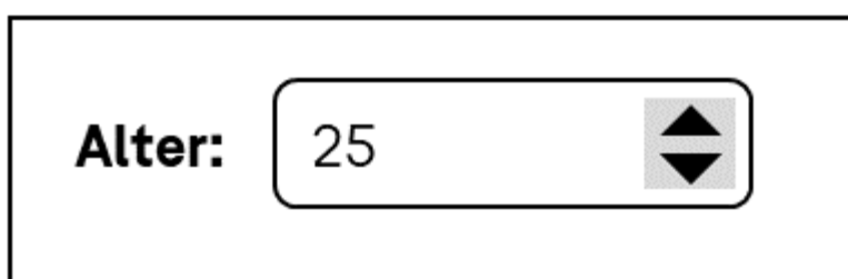
Abbildung: Drehfeld
