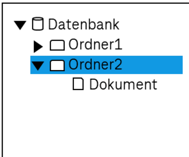
Abbildung: Baumstruktur
